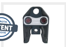
Persbekken met "E"-vormig profiel - Gepatenteerd Eurotis Mâchoire de pressage à profilé « E » - brevet Eurotis
